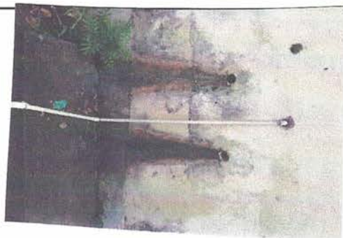
Foto 9 : Sustitución de tubería PVC línea principal aguas pluviales
