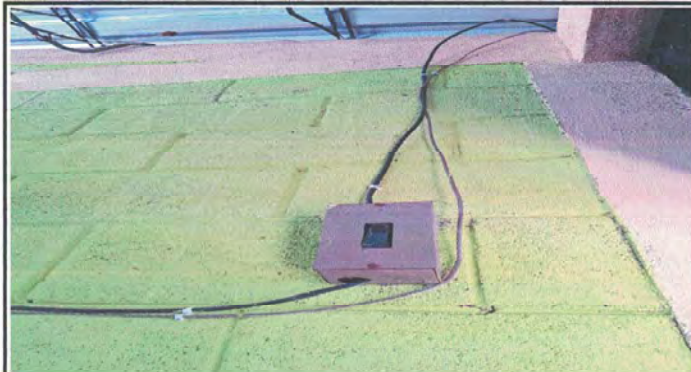
Foto 2: SISTEMA ELECTRICO INFORMAL AULA PRE PRIMARIA.
