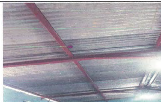
Foto 2: Sustrucción de láminas troqueladas ya que se encuentran en mal estado y con goteras.
