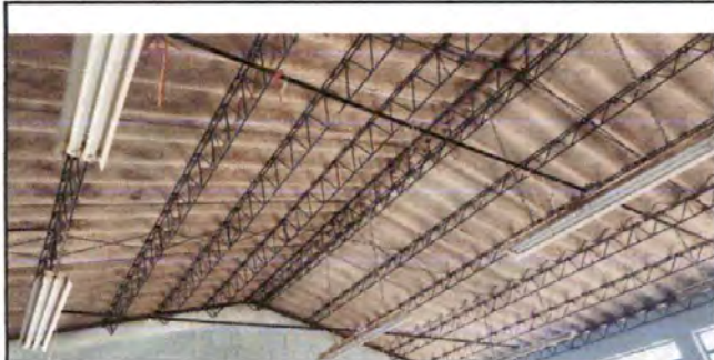
Foto 3: Vista interior de modulo 2, lamina existente de fibrocemento, se encuentra en mal estado. La estructura portante es tipo jois, necesario darle mantenimiento.
