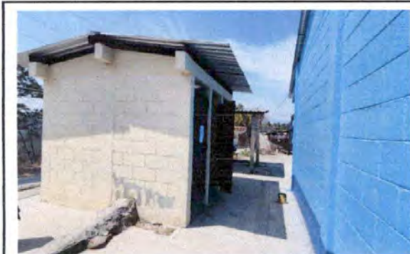
Foto 9: Vista de los baños, se necesita colocar tubería de drenaje y llevarla al fosa séptica.
