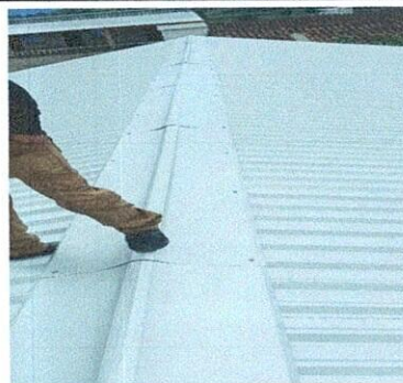
Foto 4: Finalizado del cambio de lámina, por lámina troquelada aluzinc calibre 26 y sustitución de capote de lámina para lámina troquelada.
