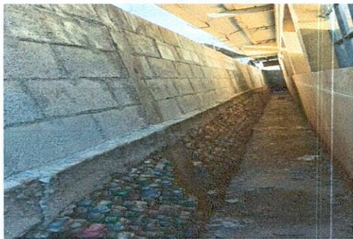
Foto 3: Proceso de reparación de muro perimetral de block y columnas.
