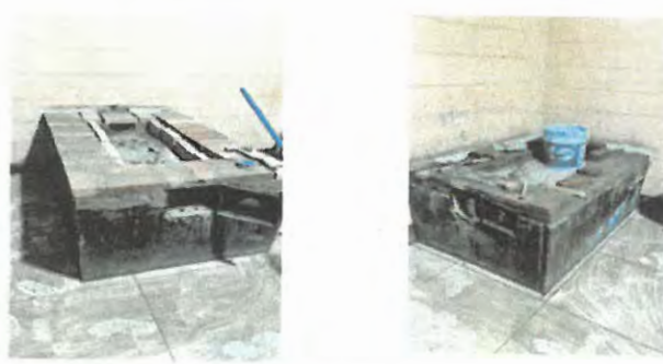
REPARACIÓN DE COCINA. Mantenimiento de estufa rural; Sustitución de plancha de metal de tres hornillas; Instalación de azulejo en estufa rural.
