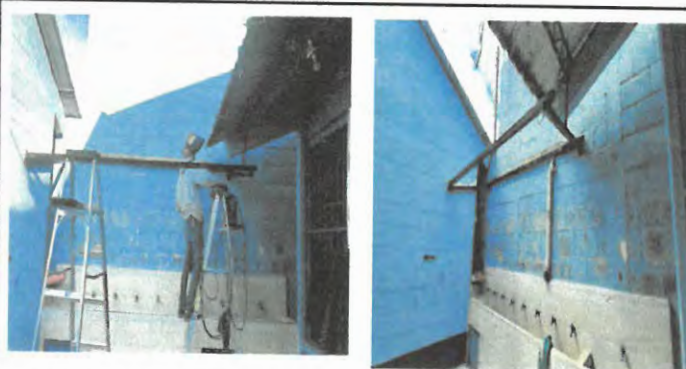
CUBIERTA DE LAMINA, Sustitución de lámina, por lámina troquelada aluzinc calibre 26. ESTRUCTURA DE TECHO, Sustitución de estructura de soporte de madera por metal.
