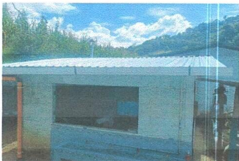
Foto 1: Área de sustitución de lamina acanalada por lamina troquelada incluye canalización de agua pluvial
