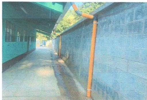
Foto 2: Aula 1 y 2 sustitución de tubo PVC por canal caudal y bajadas de agua pluvial
