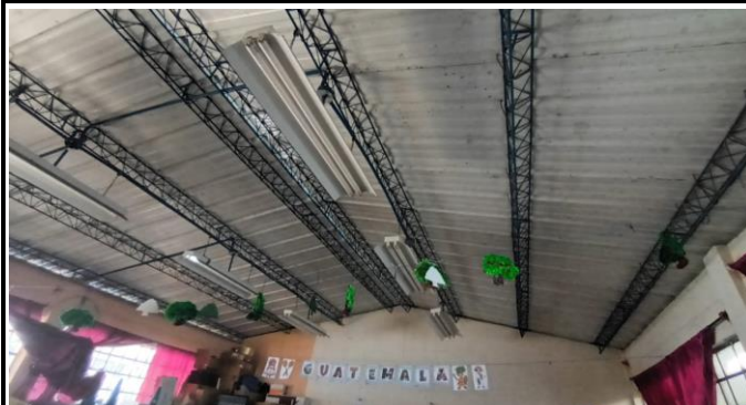
Foto 2: Techo de una de las aulas del segundo nivel donde se colocará el cielo falso de cuarto primaria.
