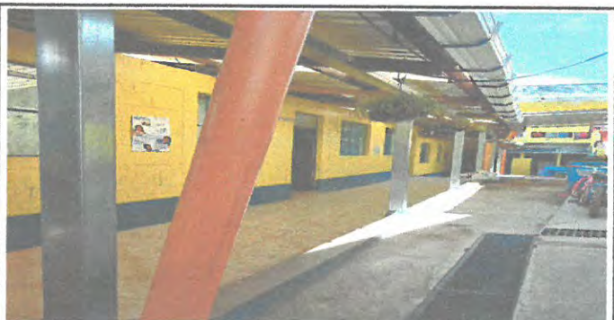
Foto 2.1 SUSTITUCION DE 6 PILARES Y UNA VIGA DE MADERA POR METAL GALVANIZADO EN CORREDOR FRENTE A TRES AULAS
