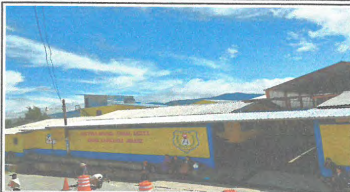
Foto1 .1: SUSTITUCION DE ESTRUCTURA DE MADERA POR ESTRUCTURA METALICA DE COSTANERAS,VIGAS Y LAMINAS TROQUELADA CALIBRE 26 EN EL PASILLO HACIA LA COCINA
