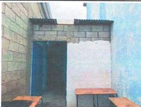
Area de sustitucion de lamina acanalada por lamina troquelada
