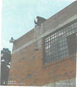
Foto 1: Echándole AGUALOK para impermeabilizar muros de ladrillos interiores y exteriores
