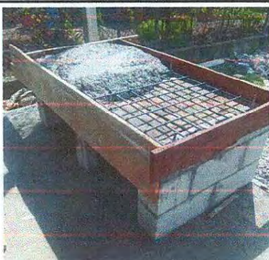
FOTO 3: SUSTITUCION DE PLANCHA DE METAL DE 3 HORNILLAS INCLUYE CHIMENEA 1.20 X 1 METRO
