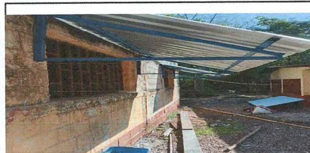
Foto 6: Sustitución de estructura de soporte de madera, por metal.
