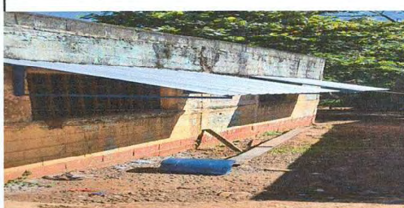
Foto 2: Sustitución de cubierta de lámina, por lámina troquelada aluzinc calibre 26
