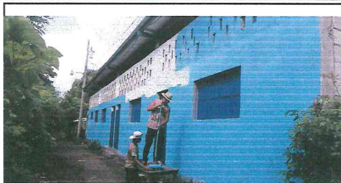
Foto 2: mantenimiento en estructura de metal de puertas, ventanas y balcones, fabricacion e instalacion de balcones de metal en ventanas. Pintura en muro exterior
