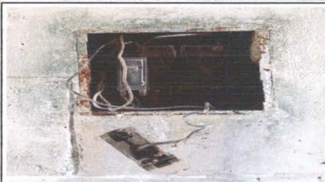
Sustitución de tomacorrientes en módulo de aulas
