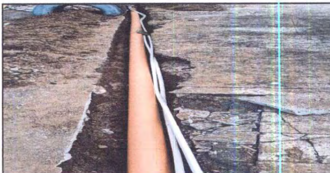
Foto 12: Sustrucción de tubería PVC línea principal aguas negras
