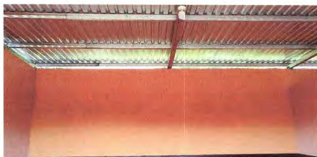
Foto 2: Aulas sustitución de estructura de soporte de madera por metal
