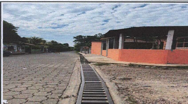
Sustitución de Malla Galvanizada por estructura de metal Módulo No. 1 Muro Perimetral
