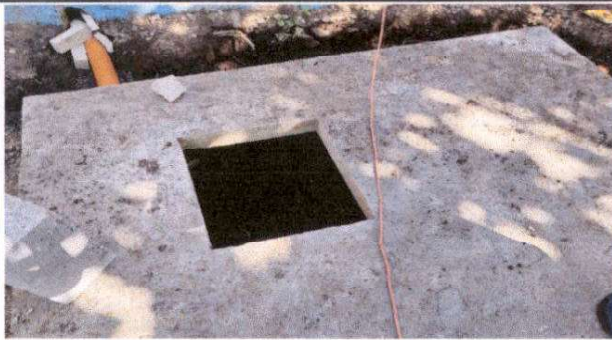
Foto 1: Sustrucción de fosa Séptica
