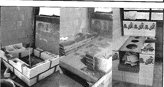
Sustitucion completa de plancha para cocina
