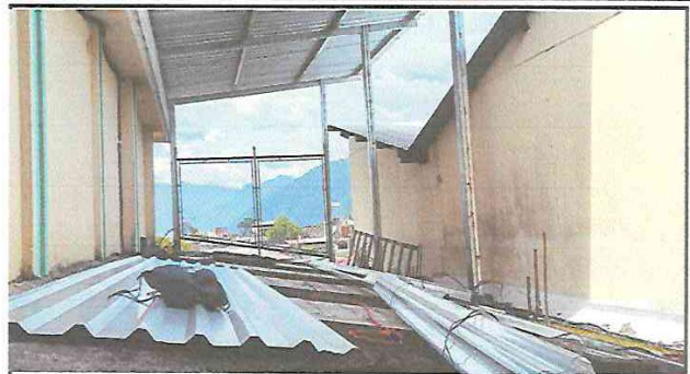
Foto 2: ESTRUCTURA DE TECHO: Fase concluida de Postes de metal y costaneras para la colocacion de lamina troquelada.
