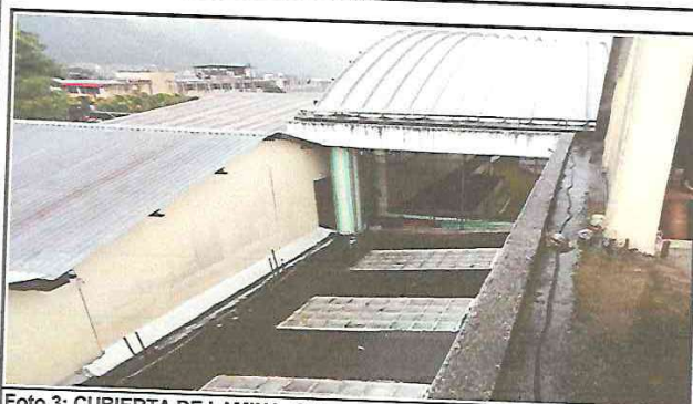
Foto 3: CUBIERTA DE LAMINA; Colocación de laminas troqueladas y lamiluz para evitar la caída de agua pluvial hacia el Establecimiento e instalación de canal de tubo plastico sobre loza para salida de aguas pluviales
