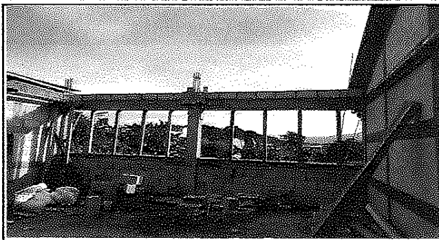
Foto 2: Avance de la sustitución del muro del aula.
