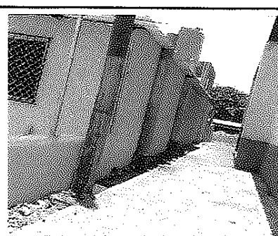
Culminación de la colocación de los tubos de chimeneas.
