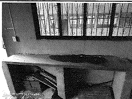
CULMINACION DE MESA DE CONCRETO DE 60 CM ANCHO X 2 MTS LARGO Y ALTURA 1 METRO ALTURA.
