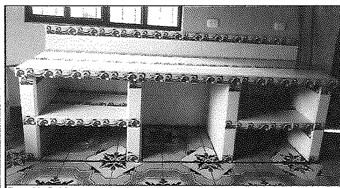
Foto 11: Gabinete terminado para la preparación de los ingredientes (cortar, pelar) y espacios para guardar los trastes.
