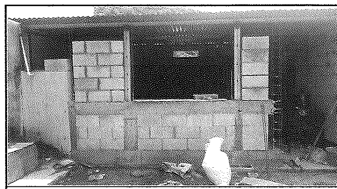
Foto 12: Levantada de pared con acceso de 1 puerta.
