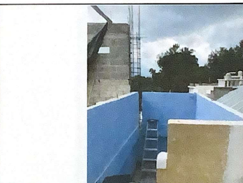
Foto 4: Colocación de techo y protección de gradas
