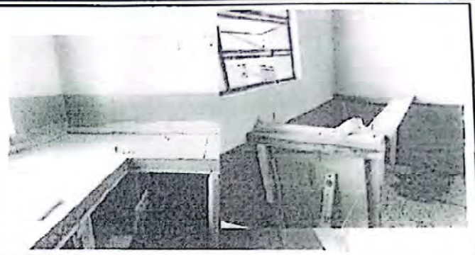
FOTO 2: Proceso de construcción de mesas de concreto armado.
