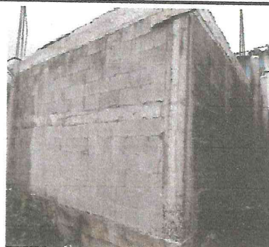
Foto 4: Reforzamiento muro perimetral con columnas y vigas de concreto.
