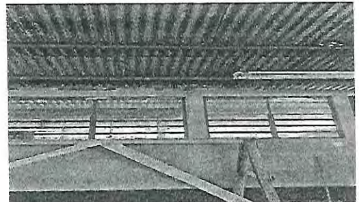
Levantado de block 1 hilada sobre solera, corona y mojinetes para sellar abertura
