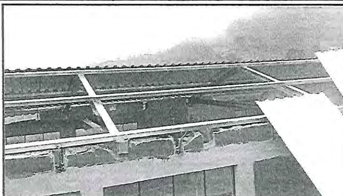
Foto 2: costaneras de metal para fijacion de laminas acanaladas
