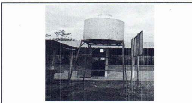
Foto 6: Se observa que la estructura está muy oxidada y picada. Se requiere de sustitución de estructura y sustitución de depósito de agua topoplast y sustitución de tubería y accesorios.
