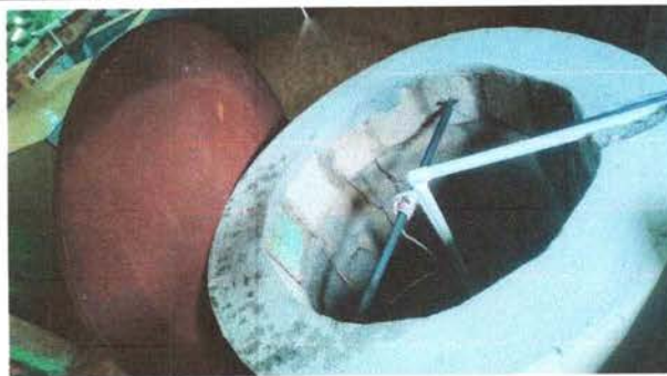
FOTO 6: Proceso de instalación de tapadera de metal en pozo de agua.
