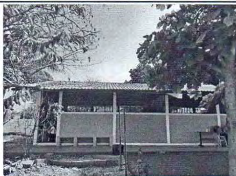
Foto 10: Se observa lámina de la cubierta existente en el módulo 2, necesita mantenimiento
