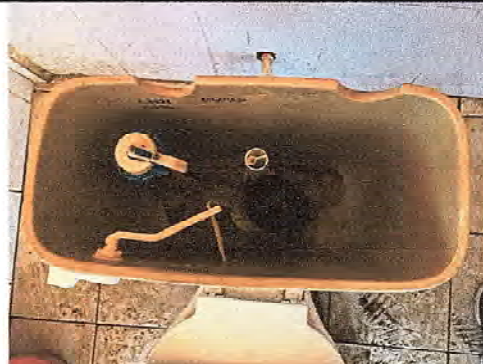
Foto 8: Se observa que sus componentes se encuentran en mal estados y ya no cumplen su funcion, y el agua tiende a filtrarse por la union del suelo y el inodoro
