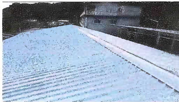
Foto 2: Módulo 1: Sustitución de lámina, por lámina troquelada aluzinc calibre 26
