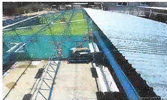
Foto 4: Modulo 1: Instalación de estructura portante de metal
