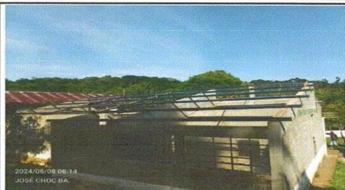
Foto 1: Sustrucción de lámina, por lamina troquelada aluzinc calibre 26
