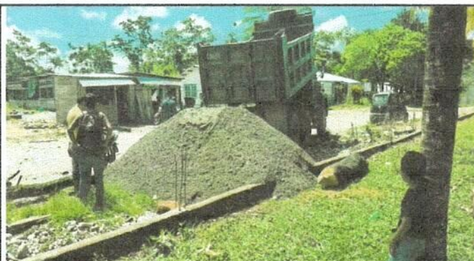
Foto 3: Reparación de muro perimetral de block con tubo hg y malla galvanizada, soleras intermedias y columnas.
