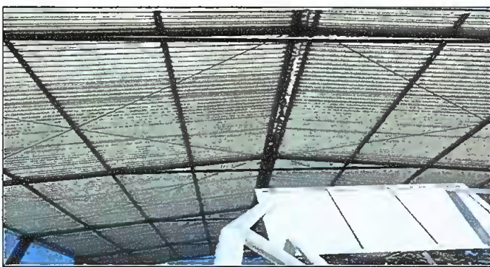
Foto 6: SUSTITUCIÓN DE ELEMENTOS DE FIJACIÓN (TORNILLOS) MODULO II.
