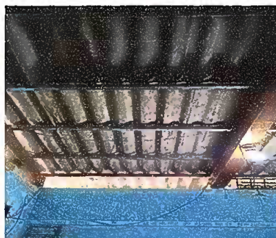
Foto 4: Estructura de techo de dirección. 1) Sustitución de lamina, por lamina troquelada aluzin 26. 2) Sustitución de estructura de madera por metal.
