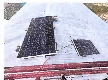
Foto 10: Modulo II: Sustitucion de panel solar 550 wts, inversor 3000 wts, baterias de 200 amp, regulador de 60 amp.
