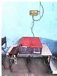
Foto 10: Modulo II: Sustitucion de panel solar 550 wts, inversor 3000 wts, baterias de 200 amp, regulador de 60 amp.
