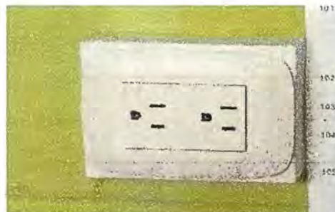
Foto 6. Módulo 3: Sustitución de tomacorrientes dobles.
