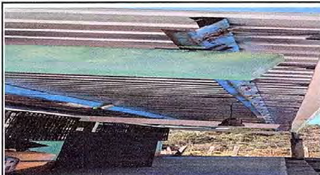
fotoграфия 3 MÓDULO 1: Sustitución de soporte o pescante de metal para canal
