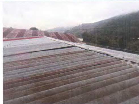
Foto 5: Lámina con agujeros, vista desde el exterior.
