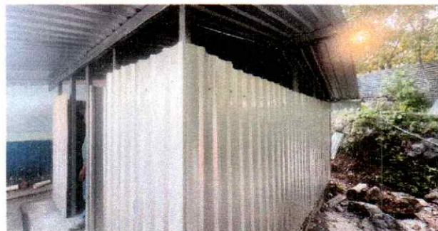
Foto 9: Se observa el avance del mejoramiento de muros, con instalación de estructura portante de metal y lámina troquelada calibre 26, en baños generales.
