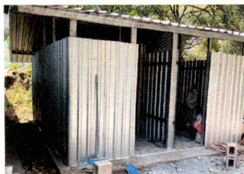
Foto 8: Se observa el mejoramiento de muros, con instalación de estructura portante de metal y lámina troquelada calibre 26 para cubierta y muros en baños generales.
