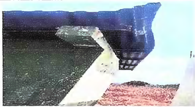
Foto 6: Desinstalacion de lamina existente e instalacion de lamina troquelada calibre 26.
