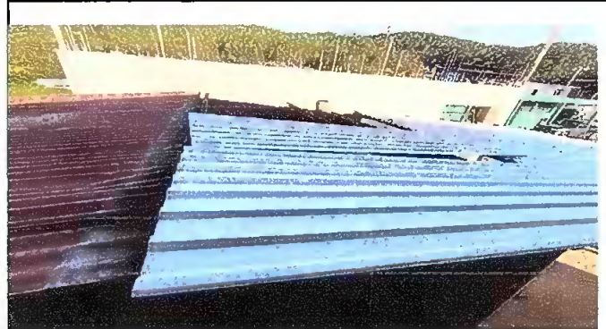
Foto 8: Desinstalacion de lamina existente e instalacion de lamina troquelada calibre 26.
