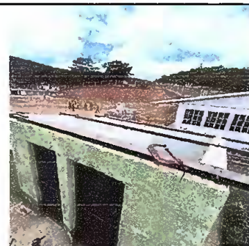
Foto 12: Desinstalacion de lamina existente e instalacion de lamina troquelada calibre 26.
