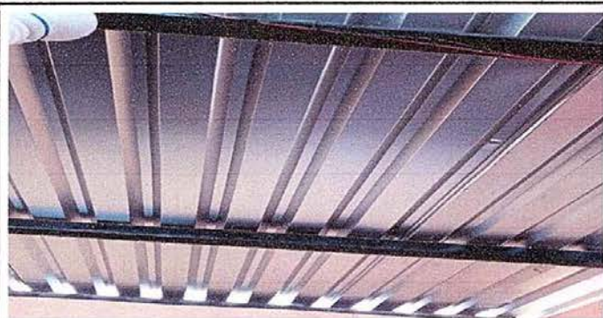
Foto 7: MÓDUO 5 Sustrución de lámina por lámina troquelada
