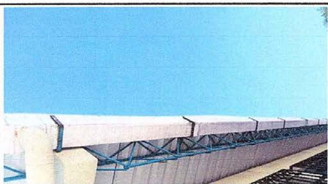
Foto 11: MÓDULO 7 Reparación de canales
